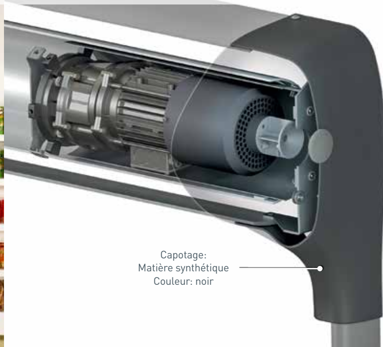
Moteur incorporé dans le tambour - DVDM PT
